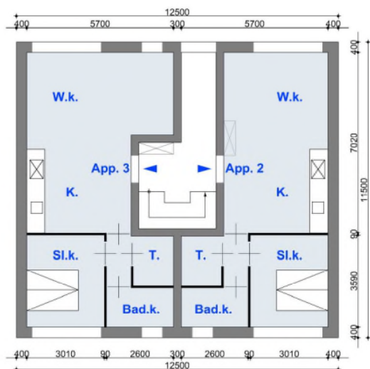
Niveau 1 Begane grond
