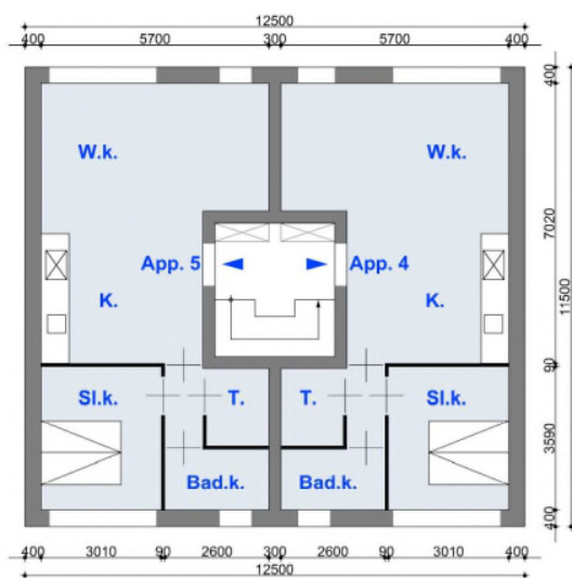
Niveau 2 1e Verdieping
